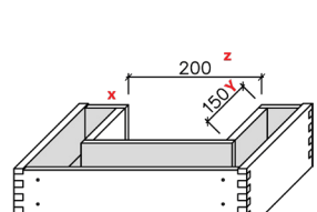
Siphonausschnitt fix 200x150 mm mittig; variabel unter der Angabe der 3 Maße x/y/z
