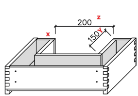
Siphonausschnitt fix 200x150 mm mittig; variabel unter der Angabe der 3 Maße x/y/z
