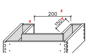
Siphonausschnitt fix 200x150 mm mittig; variabel unter der Angabe der 3 Maße x/y/z
