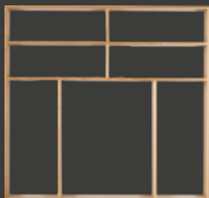
Typ U4: Höhe 52 mm oder 92 mm Tiefe 340 - 550 mm / Breite 350 - 650 mm
