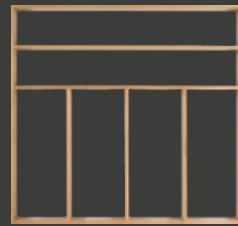
Typ U5: Höhe 52 mm oder 92 mm Tiefe 340 - 550 mm / Breite 350 - 650 mm
