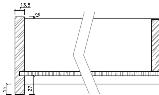
Seitenschnitt Innenlade
